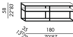
console 180/2 due ripiani - two shelves - zwei Platten deux étagères - dos estantes
