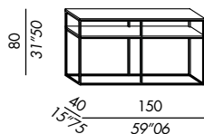
console 150/2 due ripiani - two shelves - zwei Platten deux étagères - dos estantes
